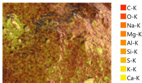
Gambar 3. Hasil Uji EDS FABA 0%.
