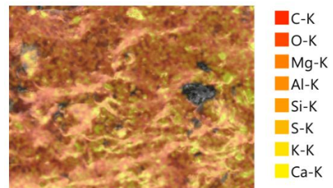
Gambar 6. Hasil Uji EDS FABA 1,5%.
