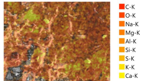
Gambar 5. Hasil Uji EDS FABA 1%.
