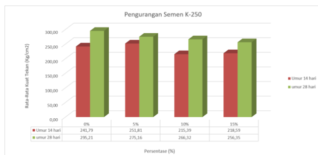
Gambar 2. Grafik Kuat Tekan Benda Uji Umur 14 dan 28 hari
